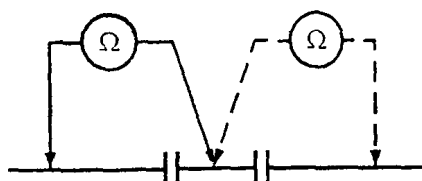
Рисунок 7. - Схема контроля состояния изолирующих фланцев с нейтральной вставкой (а) и без вставки (б)
