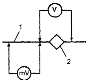
Рисунок 6. - Схема контроля состояния изолирующих муфт на кабелях приближенно без источника тока (а) и с источником тока (б)
