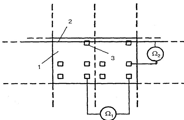
1 - блок; 2 - шина заземления; 3 - закладные детали
