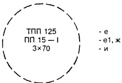
Кабели питающих линий ПП от ТПП
