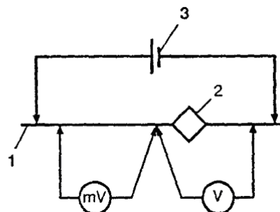
Рисунок 6. - Схема контроля состояния изолирующих муфт на кабелях приближенно без источника тока (а) и с источником тока (б)
