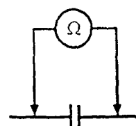
Рисунок 7. - Схема контроля состояния изолирующих фланцев с нейтральной вставкой (а) и без вставки (б)
